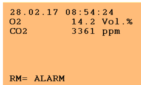
Abb. 3: Messwertanzeige
