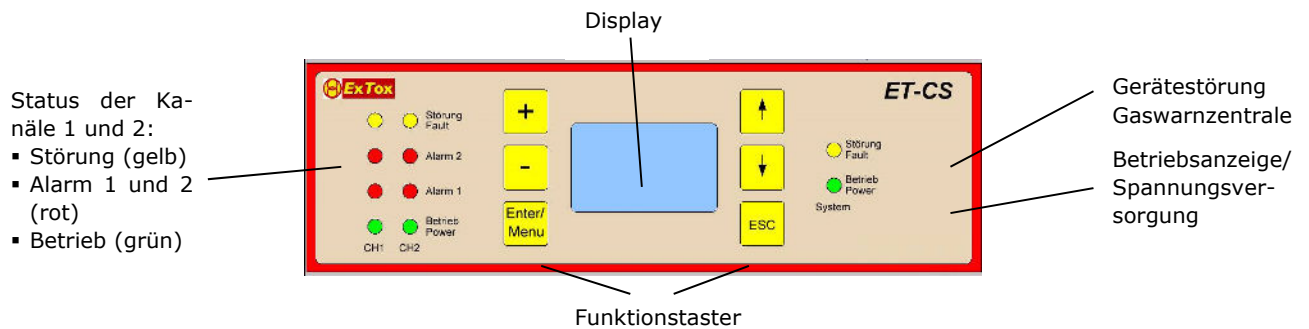
Abb. 2: Gerätepanel ET-2D
