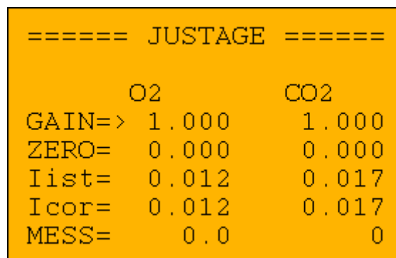
Abb. 14: Justagemenü für Analogtransmitter (Pfad: MESSWERTE > SETUP > JUSTAGE > MESSKANÄLE)
